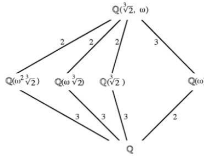
Gambar 10.1: Lattice dari Contoh 10.3.5
