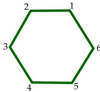
Gambar 5.1: Segi-6 beraturan
