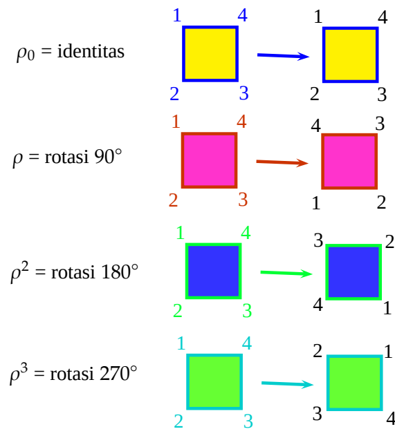
Gambar 2.2: Simetri Rotasi □
