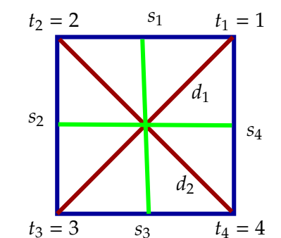
Gambar Persegi dari grup D_4 .
