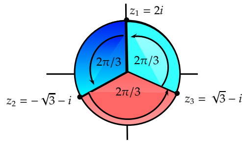
Gambar 1.9: Penyelesaian dari z^3 + 8i = 0
