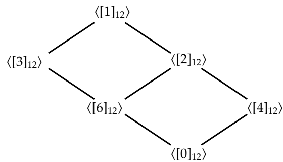
Gambar 2.5: Lattice Subgrup
