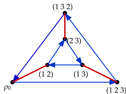
Digraf Cayley dari grup simetri S_3 dengan S = \{(1\ 2), (1\ 2\ 3)\} dan \rightarrow representasi dari (1\ 2\ 3) , sedangkan - representasi dari (1\ 2) .
