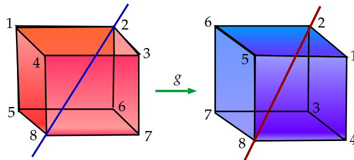
Gambar 5.2: Tindakan G pada Kubus
