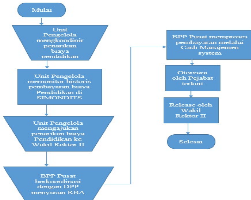
Gambar 29. Diagram alir Penarikan biaya Pendidikan mahasiswa penerima beasiswa
