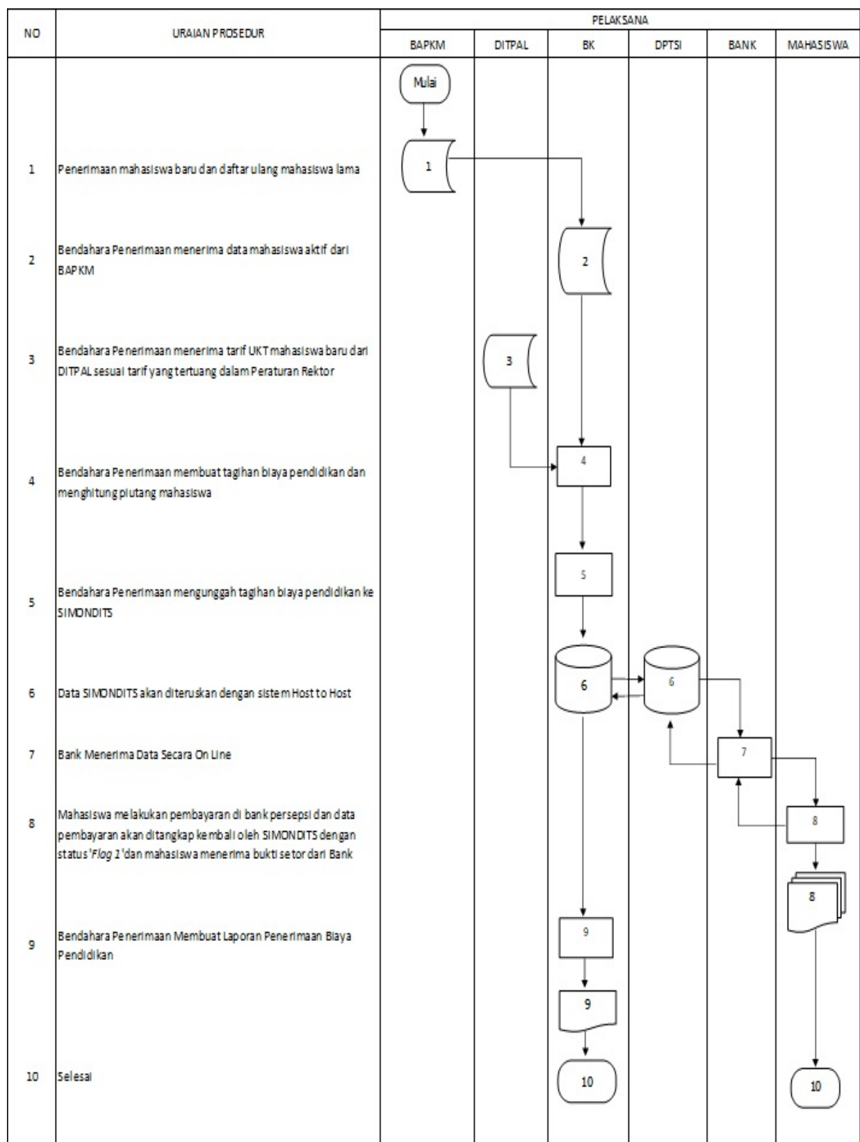
Gambar 1. Diagram Alir Penerimaan Biaya Pendidikan UKT/SPP
