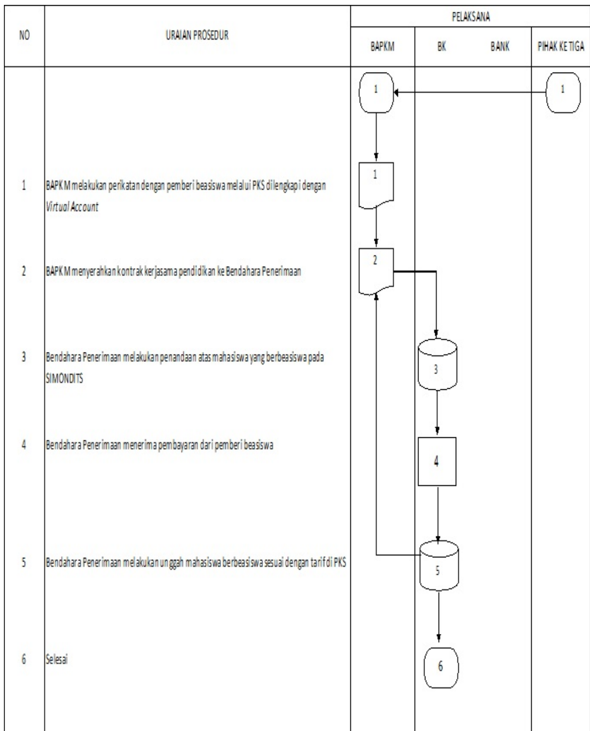
Gambar 4. Diagram Alir Realisasi Kerjasama Pendidikan
