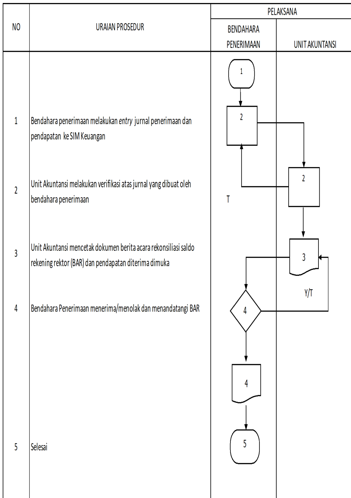
Gambar 12. Diagram Alir Rekonsiliasi Bank dan Piutang
