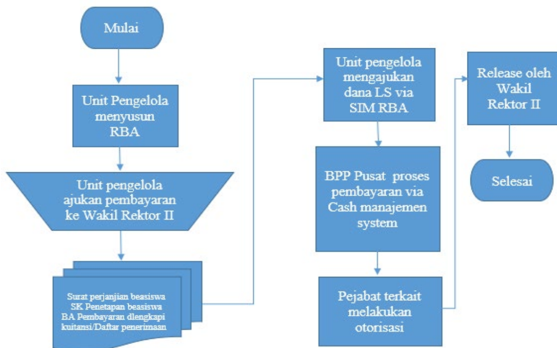
Gambar 27. Diagram alir pembayaran Beasiswa
